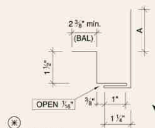
⊛ JAMB #709 (A+9"=GIRTH)
